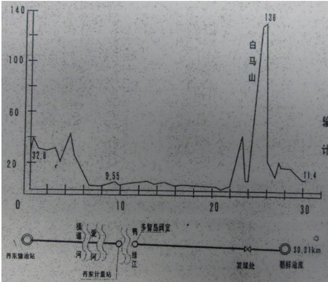
〈그림 1〉 단동-백마산 원유송유관 단면도 (단위: 해발(높이), 길이(2km))
