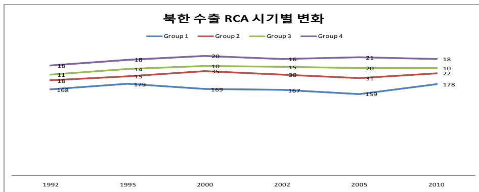
〈그림 III-5〉 북한의 수출 RCA 시기별 변화
